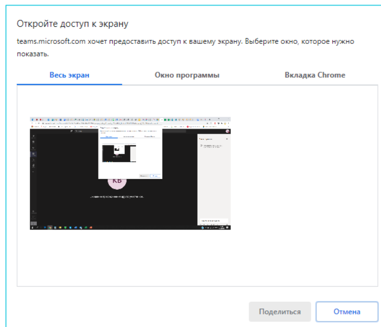
Рисунок 13. Выбор доступа
